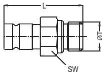
Male Threaded Shut-Off Plug Verschlussnippel mit Aussengewinde
